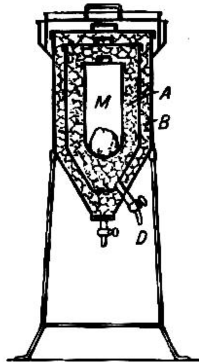
Fig. 393 Ice calorimeter (Lavoisier)
