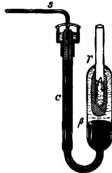
Fig. 394 Ice calorimeter (Bunsen)
